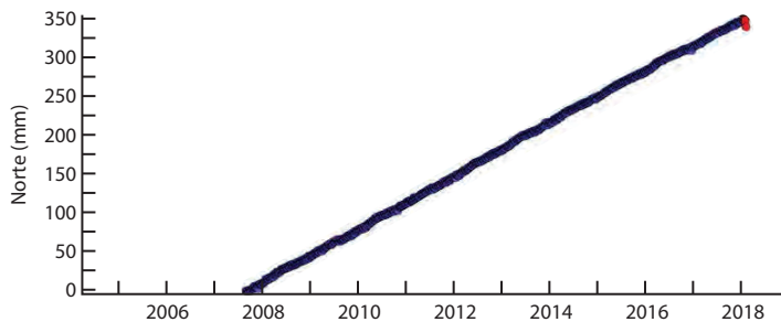
Gráfica de serie temporal de GPS para la estación AC43
