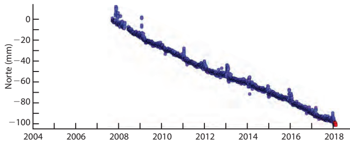
Gráfica de serie temporal de GPS para la estación AC51
